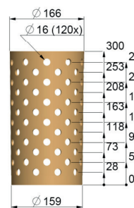
50793010 Ställbar inre ring 300 mm hög
