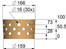
50793008 Ställbar inre ring 100 mm hög
