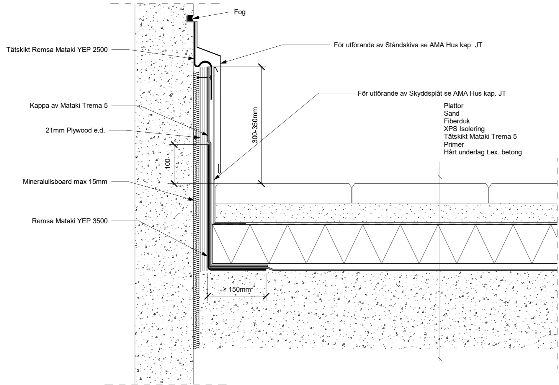
ANSLUTNING TILL VERTIKAL YTA (RÖRELSEFOG MAX 15 mm)
