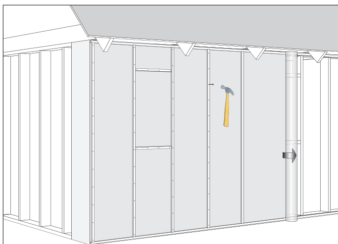
Horisontellt montage
