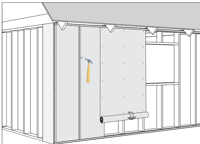
Vertikalt montage
