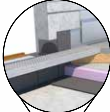
Anslutning till vertikal yta vid tröskel
