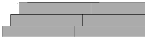
Minst 500 mm förskjutna skarvar.
